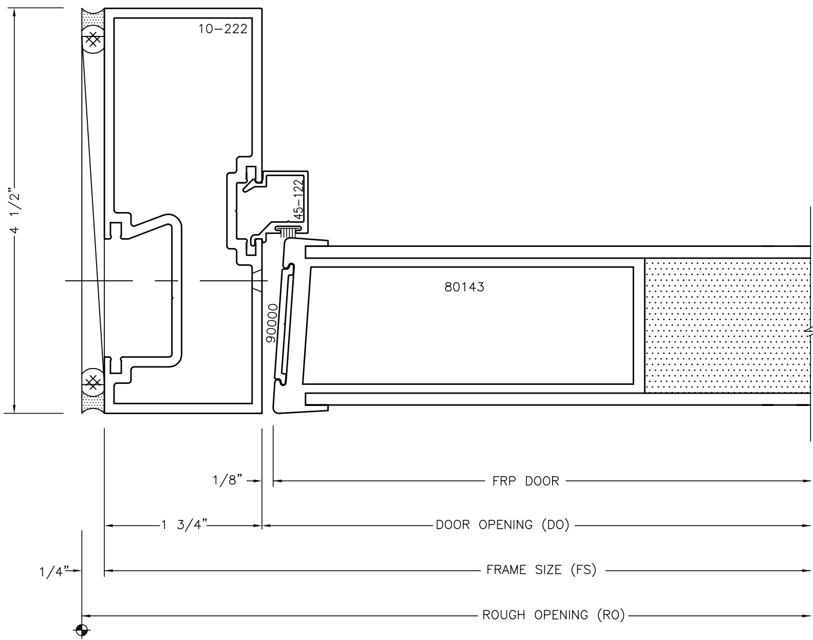
JAMB SCALE: (1=1) "
