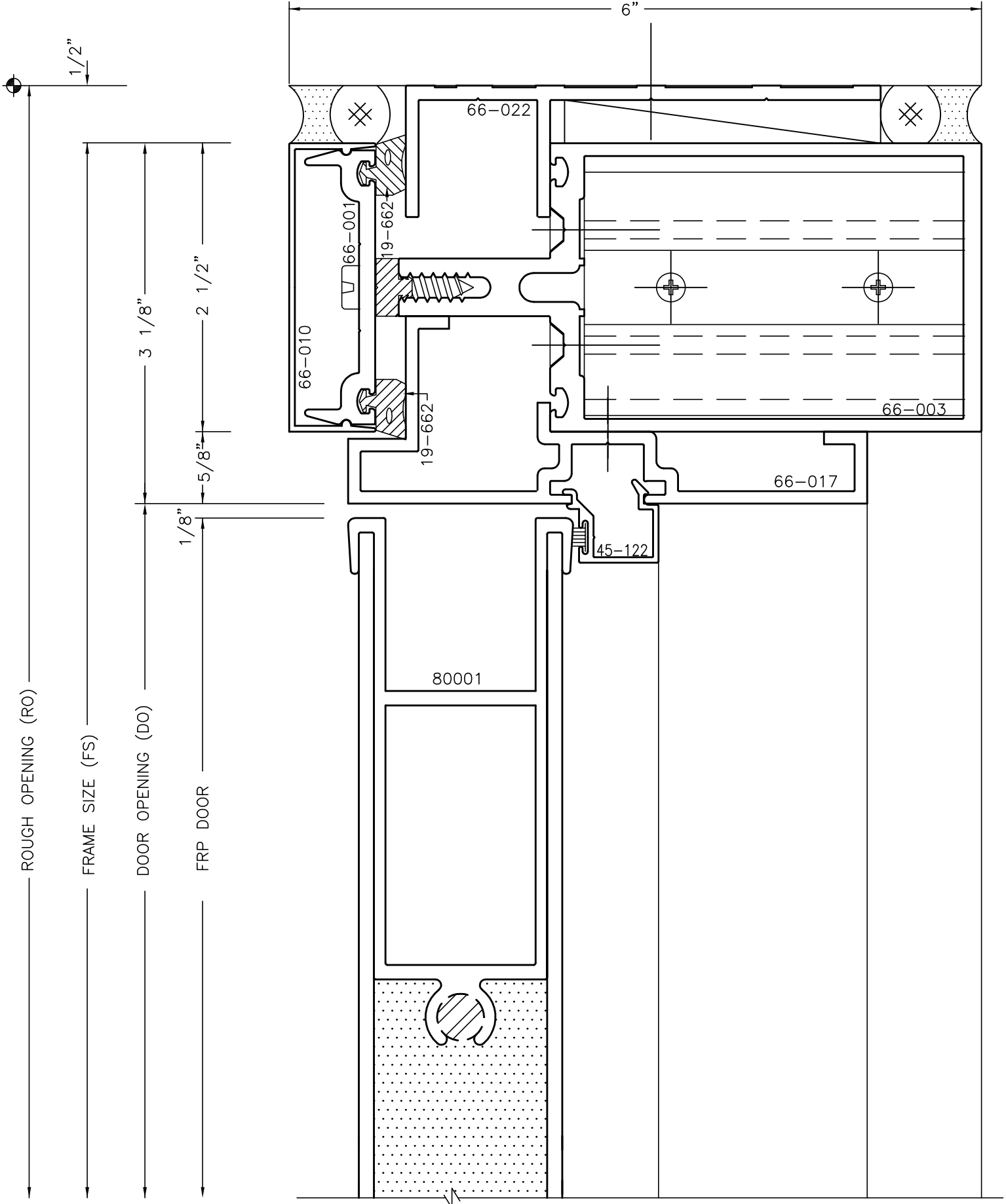
HEAD SCALE: (1=1)
