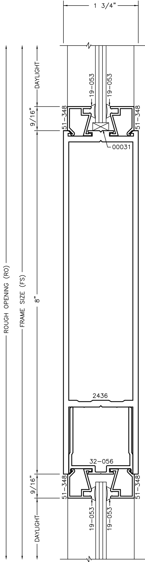
8" INTERMEDIATE CROSSRAIL SCALE: (1=1)
